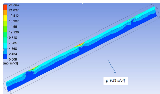
Рис. 2. Концентрация водорода на момент времени 30 секунд (моль/м³)
