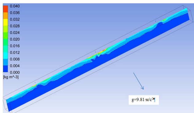
Рис. 5. Массовая концентрация водорода на момент времени 15 секунд
