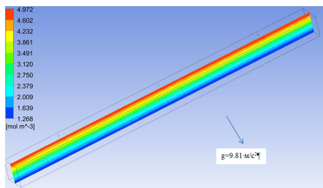
Рис. 3. Концентрация водорода на момент времени 80 секунд
