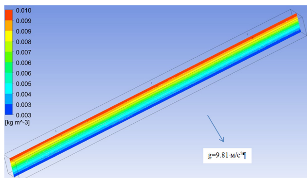
Рис. 7. Массовая концентрация водорода на момент времени 80 секунд
