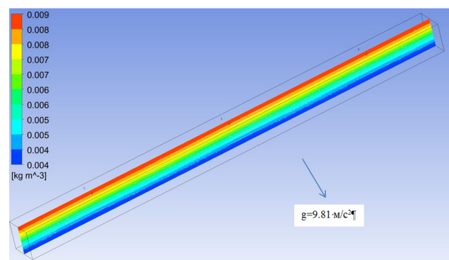
Рис. 8. Массовая концентрация водорода на момент времени 130 секунд
