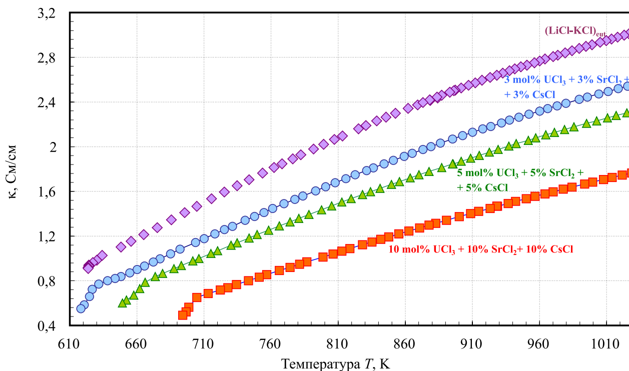
Рис. 2. Электропроводность расплавленных смесей UCl_3 и SrCl_2 с (LiCl-KCl)_{эвт} .
