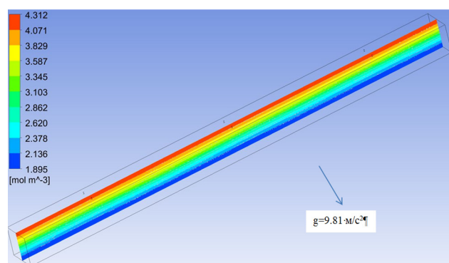
Рис. 4. Концентрация водорода на момент времени 130 секунд
