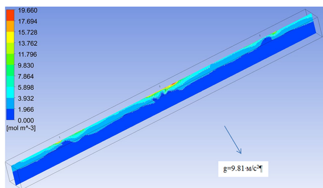
Рис. 1. Концентрация водорода на момент времени 15 секунд
