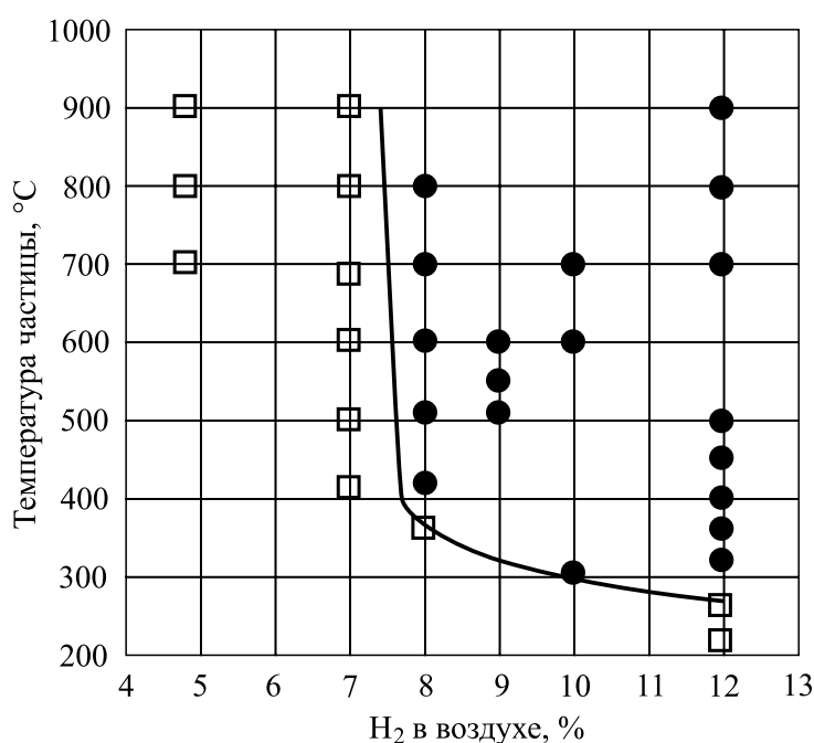
Рисунок. Воспламенение водородно-воздушной смеси при комнатной температуре нагретой каталитической частицей.
