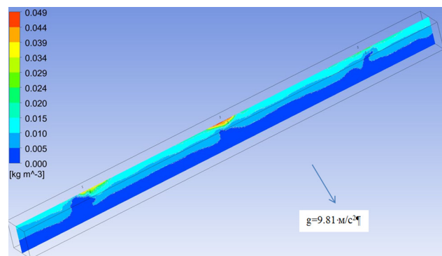
Рис. 6. Массовая концентрация водорода на момент времени 30 секунд
