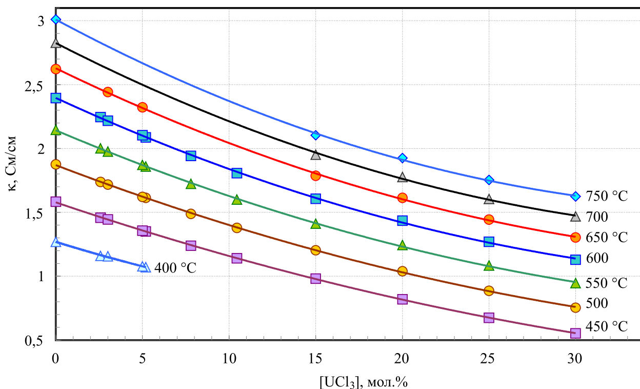
Рис. 1. Электропроводность расплавленных смесей \text{UCl}_3 - (\text{LiCl–KCl})_{\text{эвт.}} .
