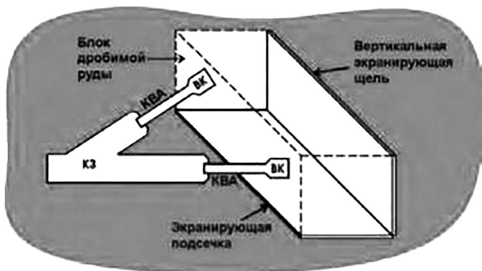
Рис. 2. Схема эксперимента «Днепр-2»
