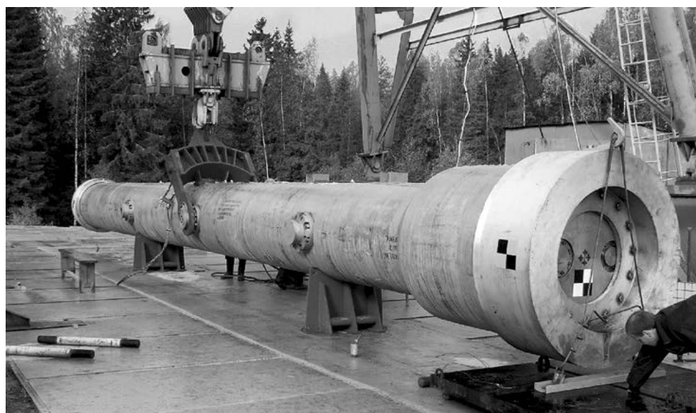
Транспортный упаковочный контейнер для хранения и перевозки отработавшего ядерного топлива
