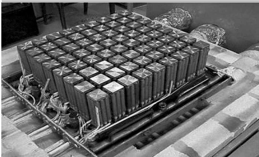
Блок батарей для твердооксидного топливного элемента
